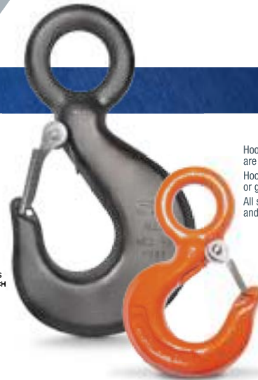
2 ton WLL & 45 ton WLL hooks shown.
